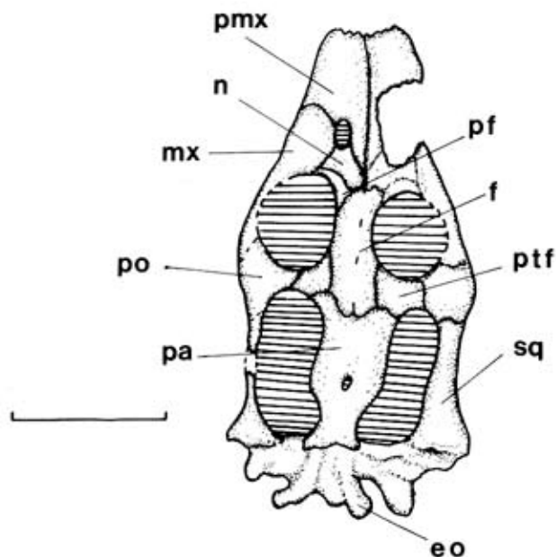
Fig. 1 - The skull of specimen 550 MCSNIO. Abbreviations: eo) exooccipital; f) frontal; mx) maxilla; n) nasal; pa) parietal; pf) prefrontal; pmx) premaxilla; po) postorbital; ptf) postfrontal; sq) squamosal. Scale bar equals 1 cm.
